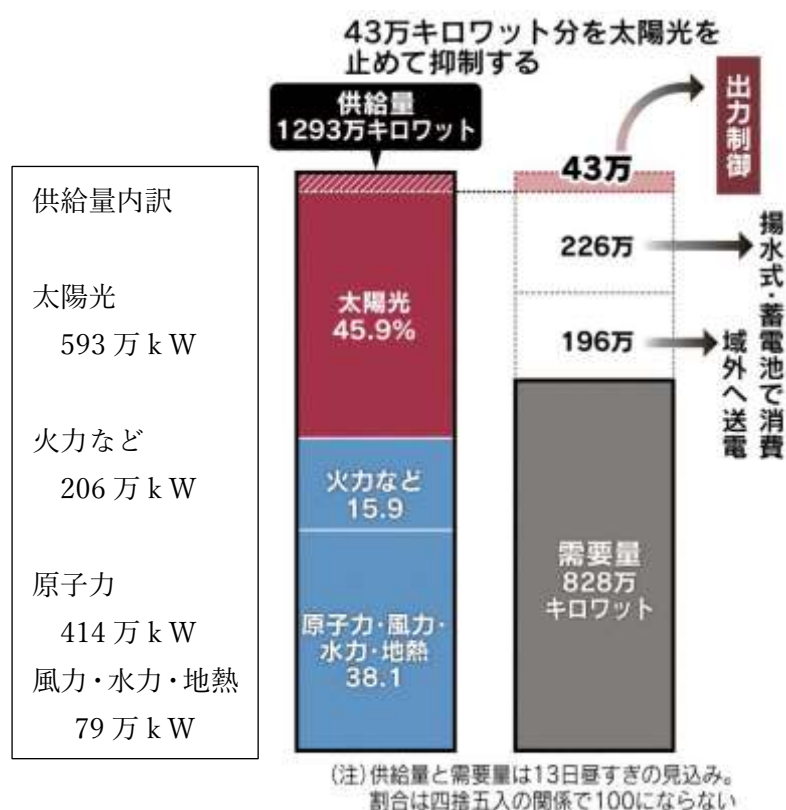
図1. 九州電力の10月13日昼過ぎにおける供給量と需要量 1
