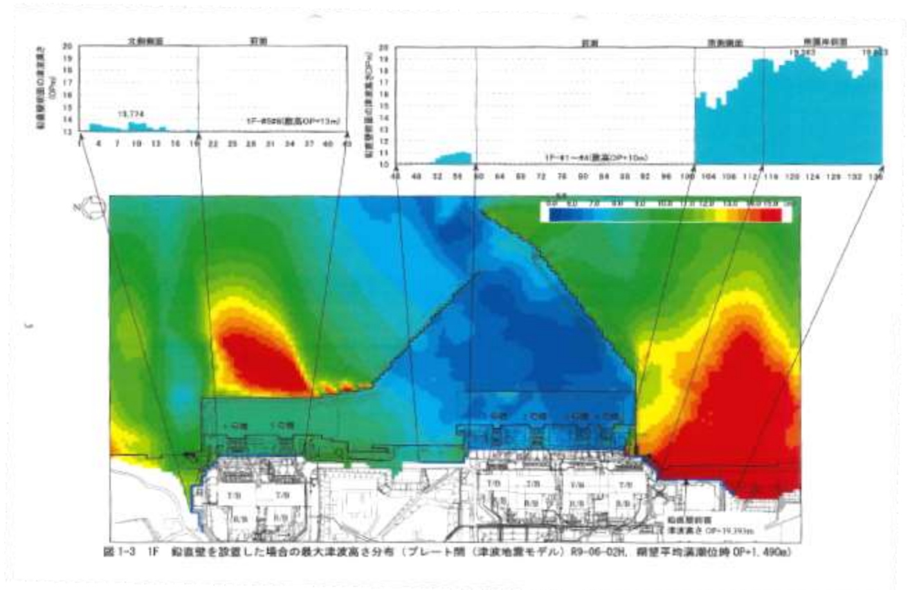
図1. 東電設計が2008年4月の報告書に記載した津波高さ予測図 図の左方向が北側を示す。
